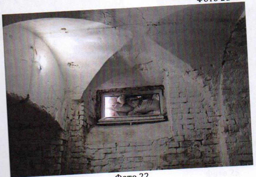
Тріщини та пошкодження опорядження стін в інтер'єрі
