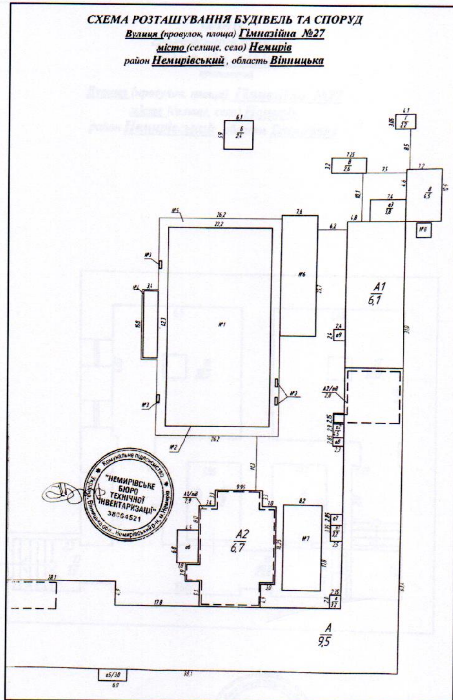
Схема розташування будівлі-пам'ятки архітектури національного значення «Чоловічий корпус» (охоронний № 976/1) комплексу споруд «Колишньої Немирівської гімназії» пам'ятки архітектури національного значення (охоронний № 976) на території земельної ділянки площею 0,4957 га
