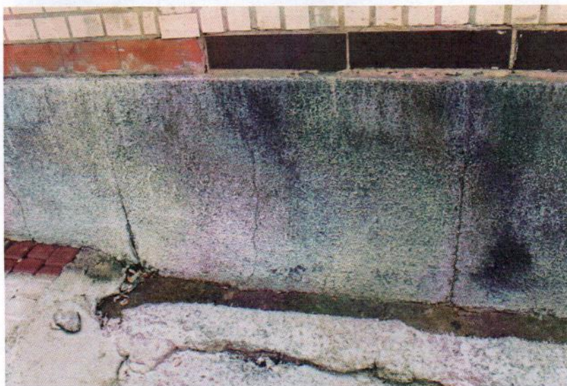
Фото 1. Головний фасад. Ділянка замокання, тріщини.
