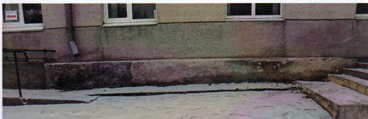
Фото 11. Вигляд дворово фасаду. Пошкодження цоколю та стіни.
