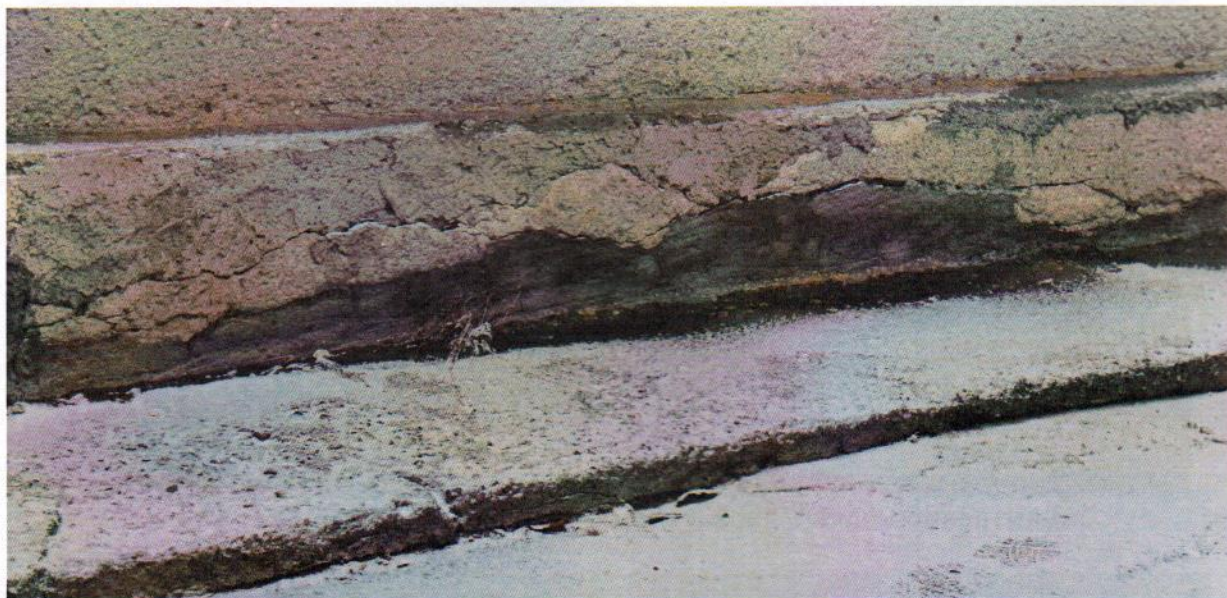
Фото 9. Вигляд дворового фасаду. Пошкодження цоколю.
