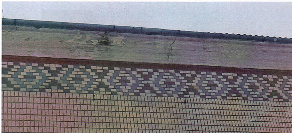
Фото 12. Пошкодження карнизу фасаду з боку пров. Кооперативний.
