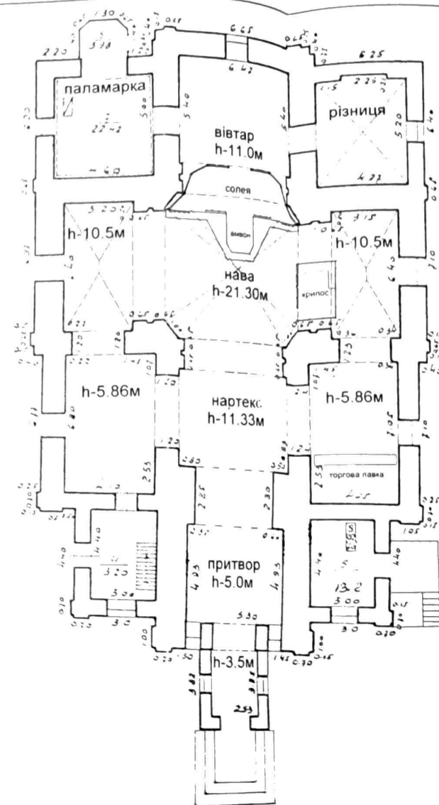
План церкви
